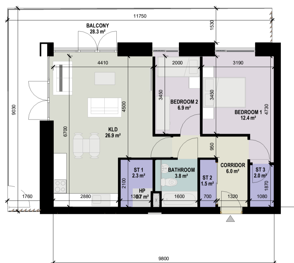
6 2BedApt_3Per_Type6 1 : 100
