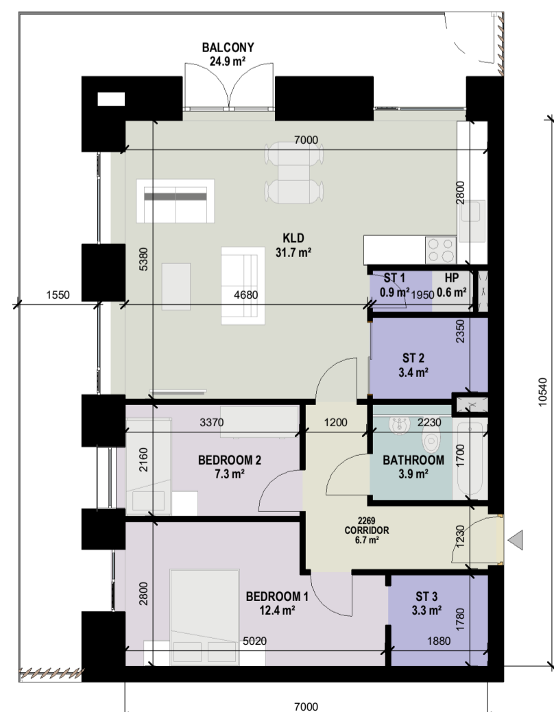
11 2BedApt_3Per_Type11 1 : 100
