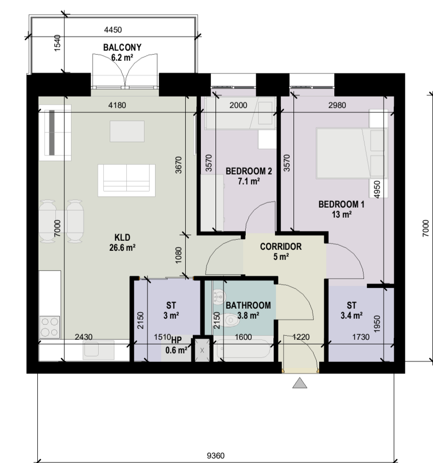
12 2BedApt_3Per_Type12 1 : 100
