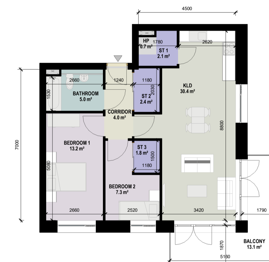
8 2BedApt_3Per_Type8 1 : 100
