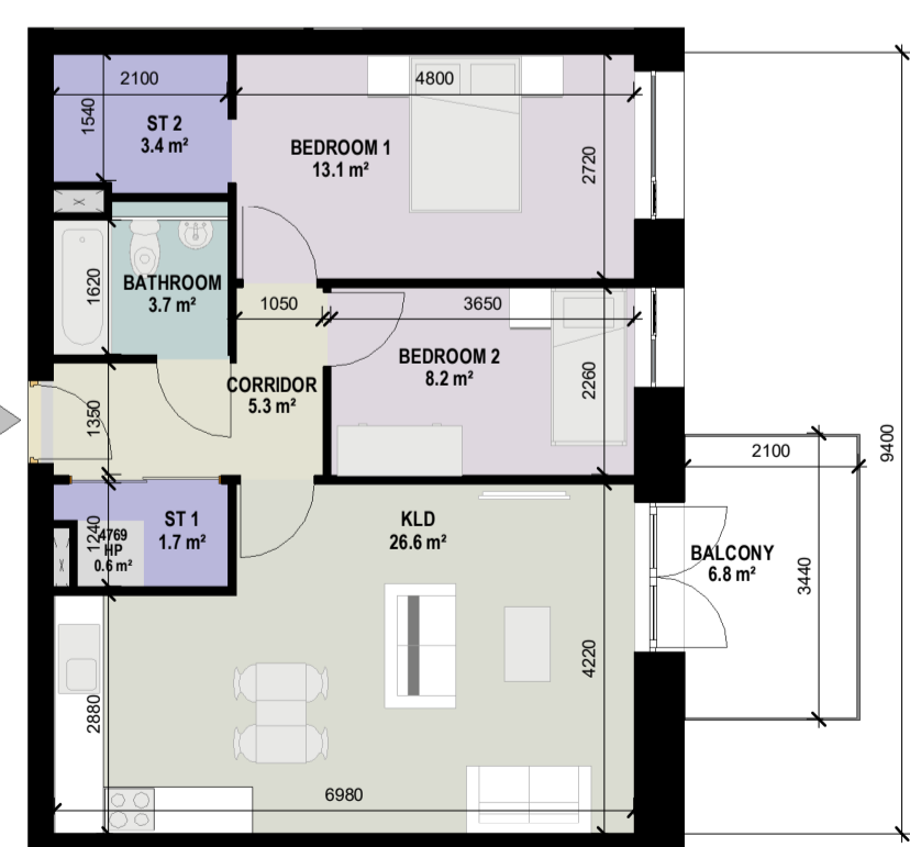
9 2BedApt_3Per_Type9 1 : 100
