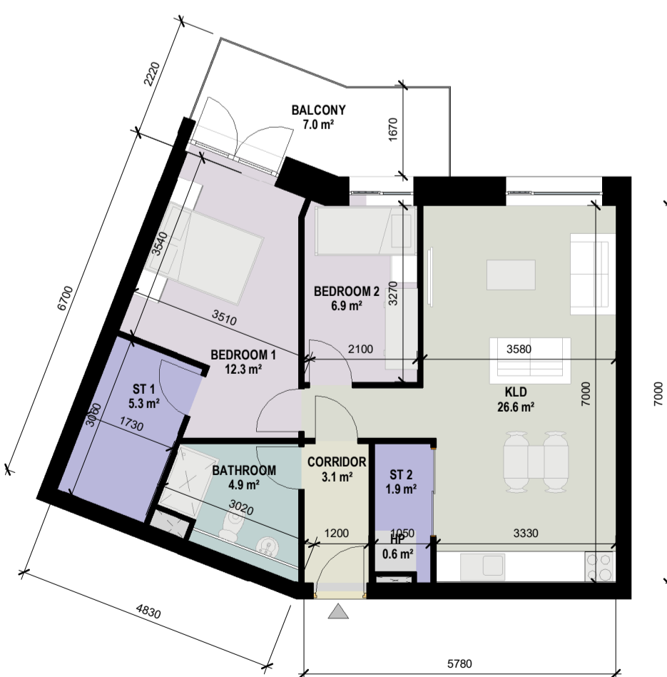
10 2BedApt_3Per_Type10 1 : 100
