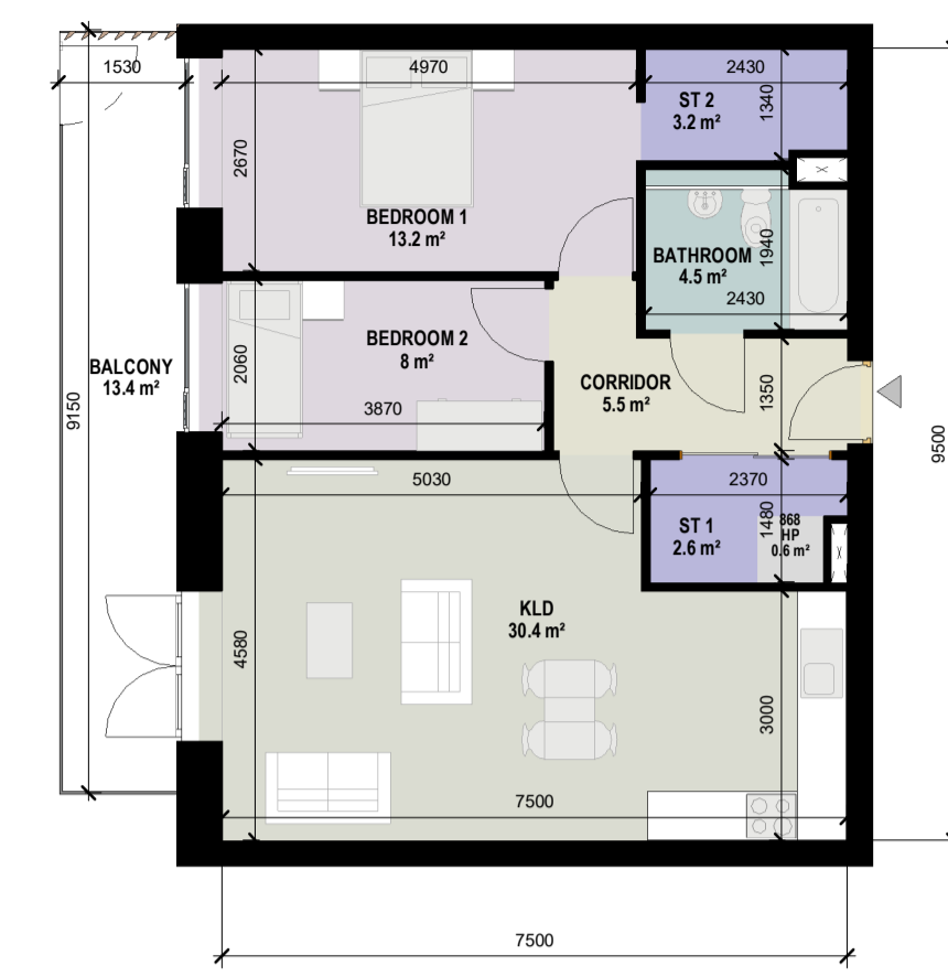
4 2BedApt_3Per_Type4 1 : 100
