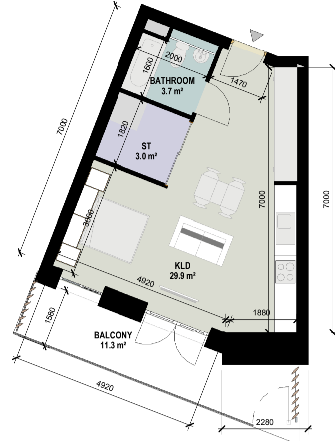
2 Studio_2Per_Type2
