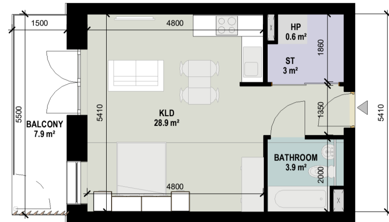
1 Studio_2Per_Type1
