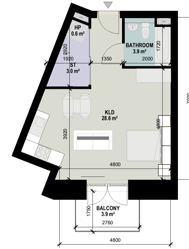
3 Studio_2Per_Type3
